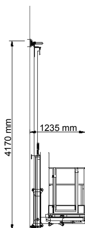
WALL-MAN® 1200 Altura padrão elevação lateral
