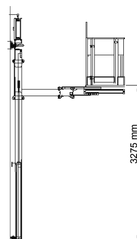
WALL-MAN® 1200 Altura padrão elevação lateral
