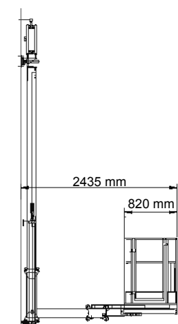
WALL-MAN® 1200 Altura padrão elevação lateral
