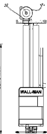
WALL-MAN® 1200 Altura estándar Elevación frontal
