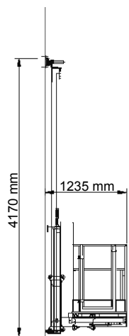
WALL-MAN® 1200 Altura estándar Elevación lateral
