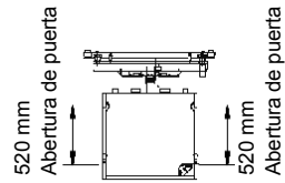
WALL-MAN® 1200 Vista plana a nivel elevado
