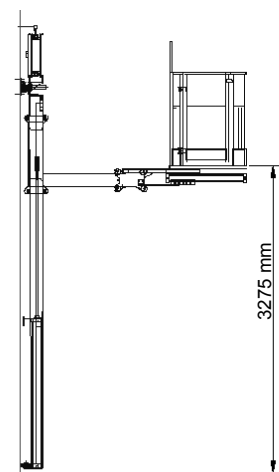
WALL-MAN® 1200 Altura estándar Elevación lateral
