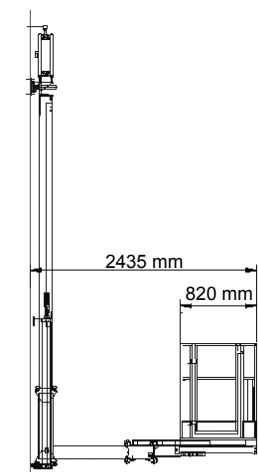
WALL-MAN® 1200 Altura estándar Elevación lateral
