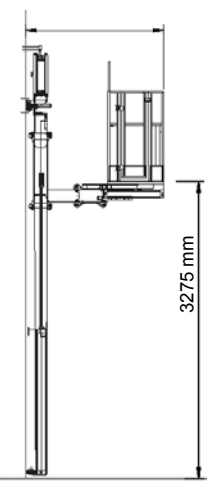
WALL-MAN® 600 Altura estándar Elevación lateral
