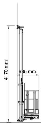
WALL-MAN® 600 Altura estándar Elevación lateral
