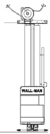
WALL-MAN® 600 Altura estándar Elevación frontal
