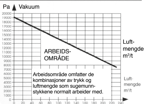
Trykkfallsdiagram
